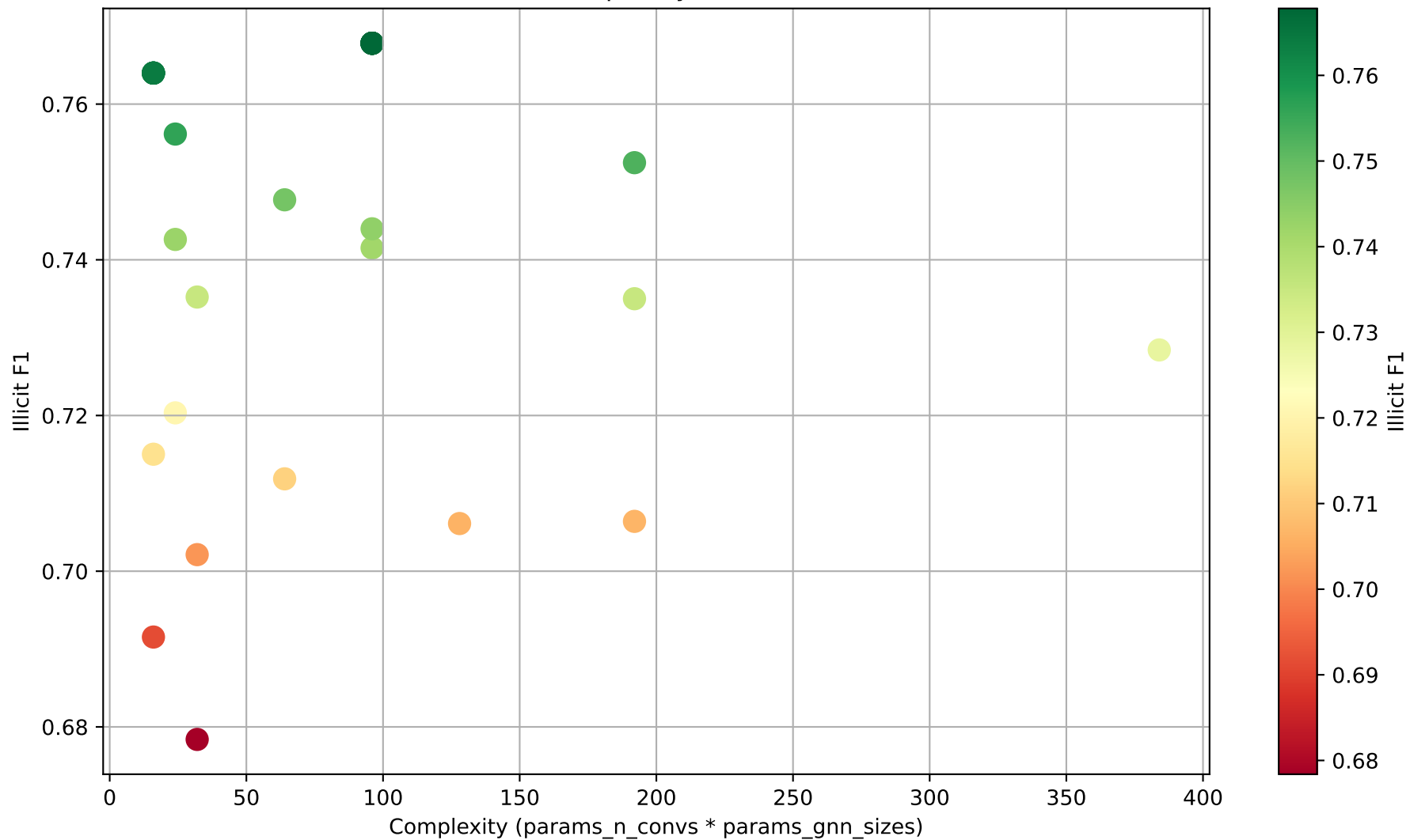
Illicit F1 vs Complexity for AMLSim 1/20
